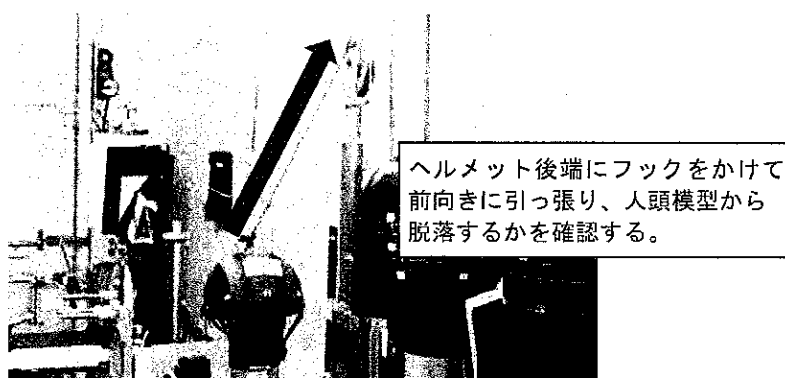
写真 3. 保持装置の性能試験の様子
