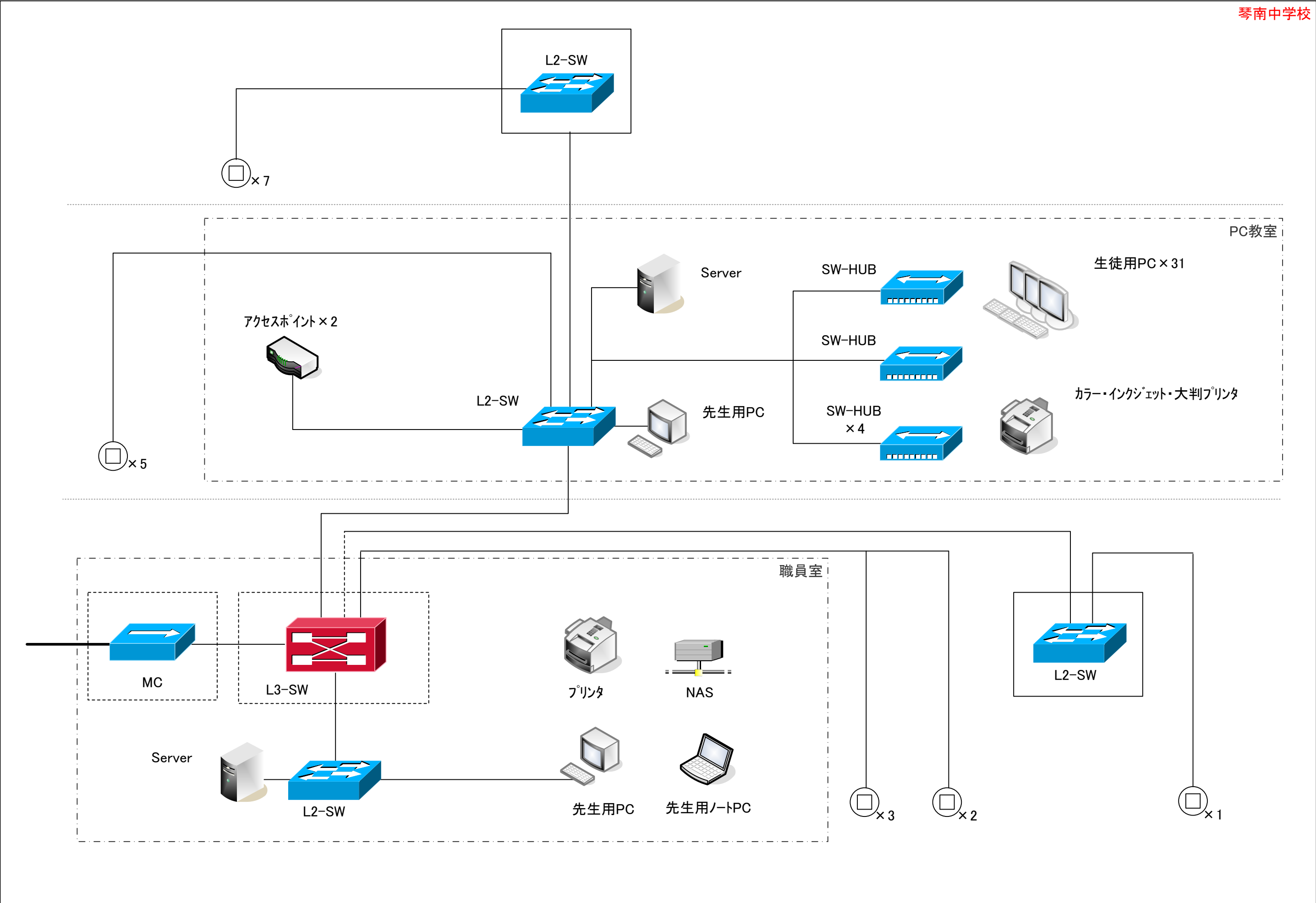
学校ネットワーク構成図(琴南中学校)
