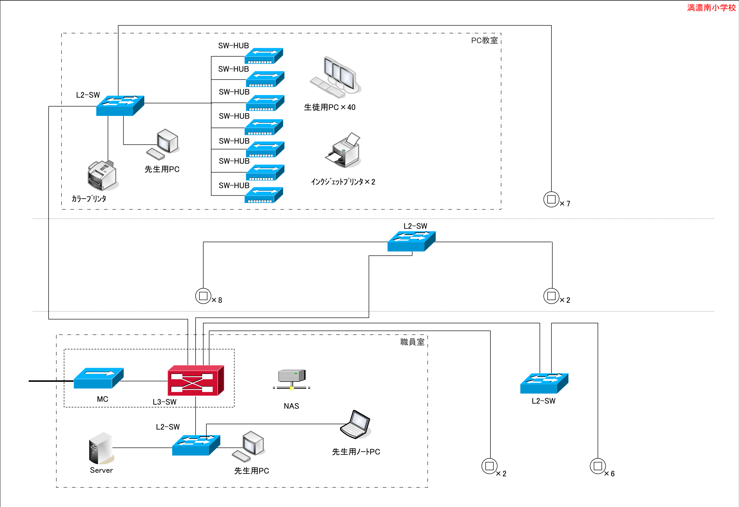
学校ネットワーク構成図(満濃南小学校)
