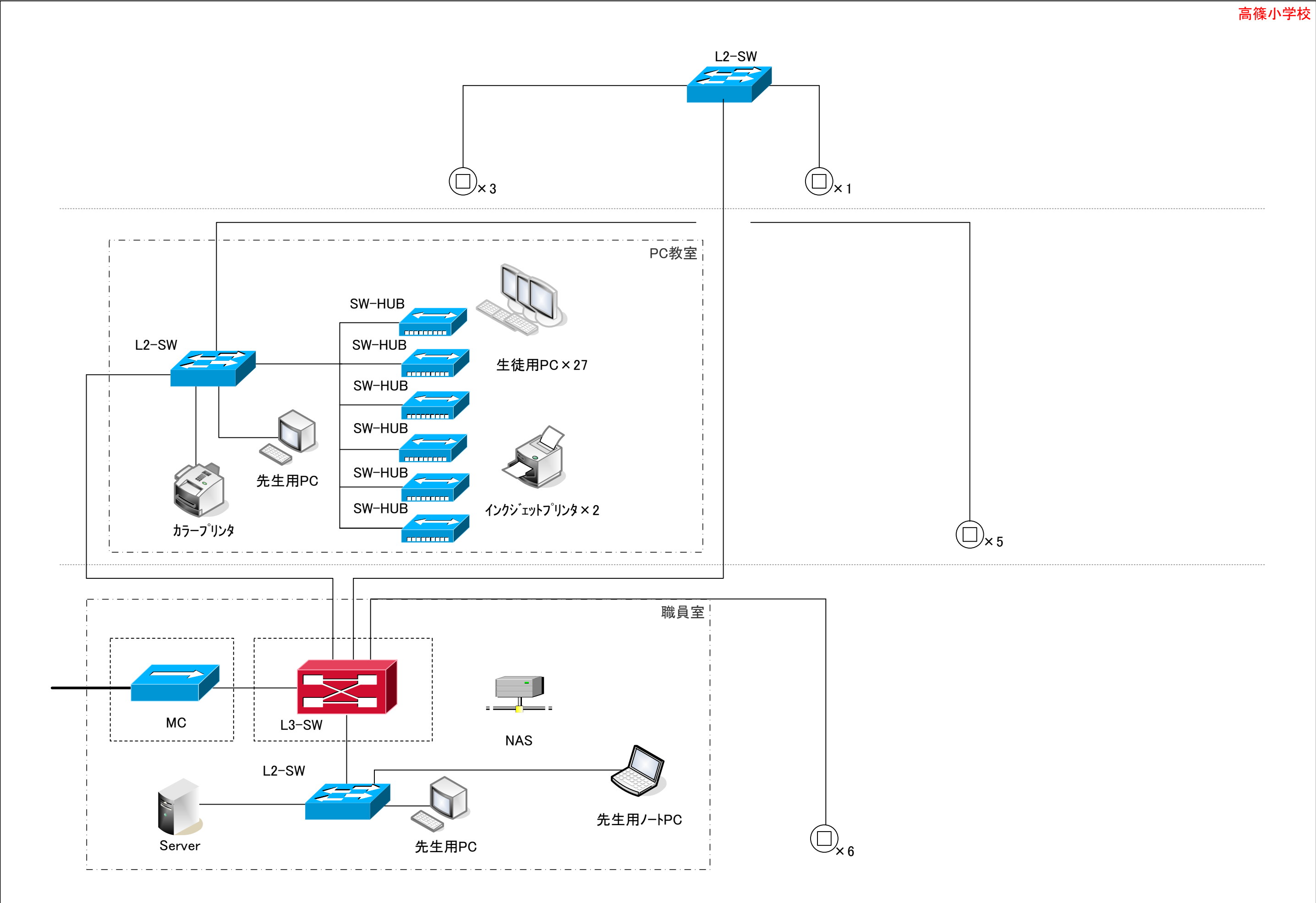
学校ネットワーク構成図(高篠小学校)
